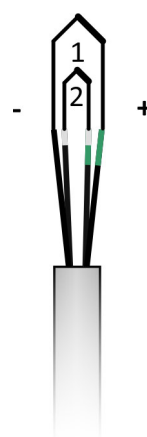
Obrázek 10.7: Zapojení dvojitého termočláneku
