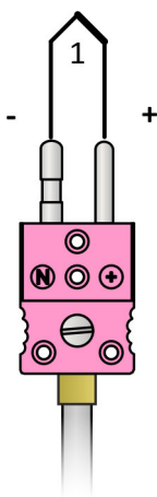
Obrázek 10.8: Zapojení konektoru
