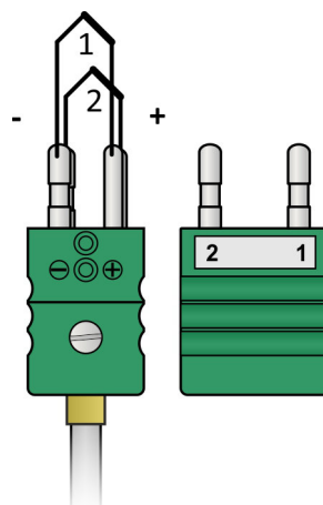
Obrázek 10.9: Zapojení dvojitého konektoru
