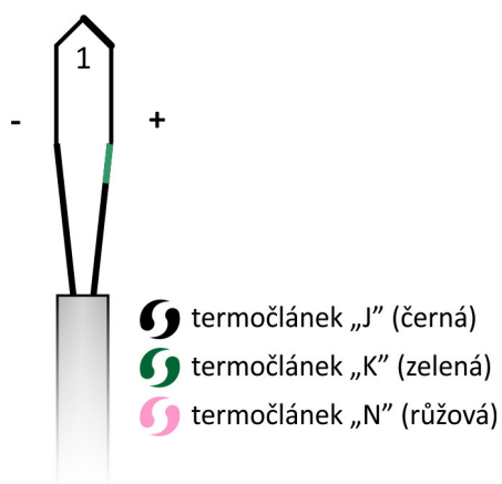
Obrázek 10.6: Zapojení jednoduchého termočláneku
